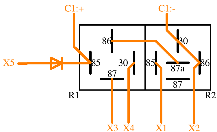
Anschlussplan Hella-Relais
