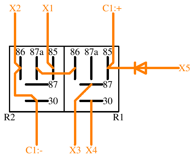
Anschlussplan MRS-Relais
